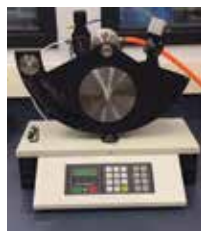
Elmendorf Tear
